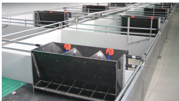
Стойловое содержание при дорастивании поросят с DryFeeder
